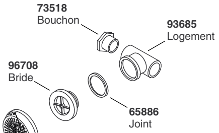
96895** (Finitions colorées) 65061** (Finitions métalliques) Couvercle
